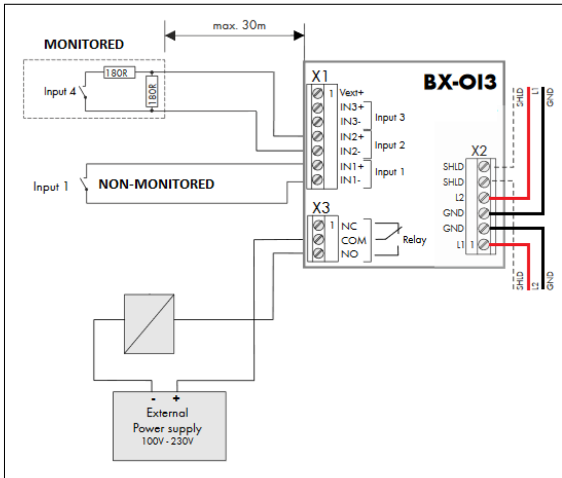
MODUL BX-OI3
