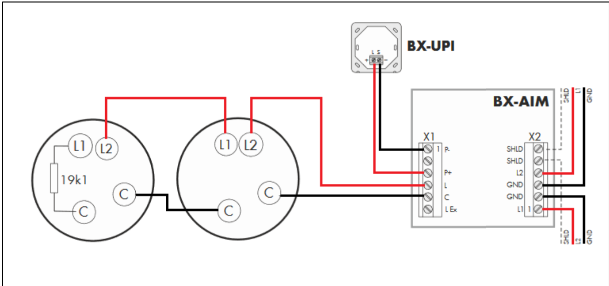
MODUL BX-AIM
