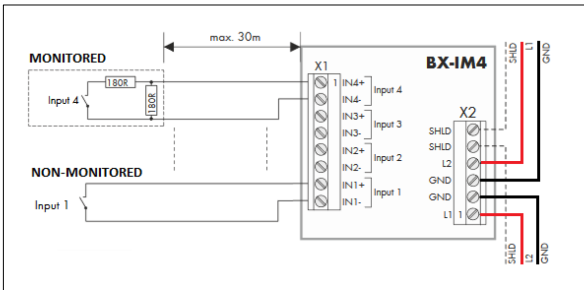
MODUL BX-IM4
