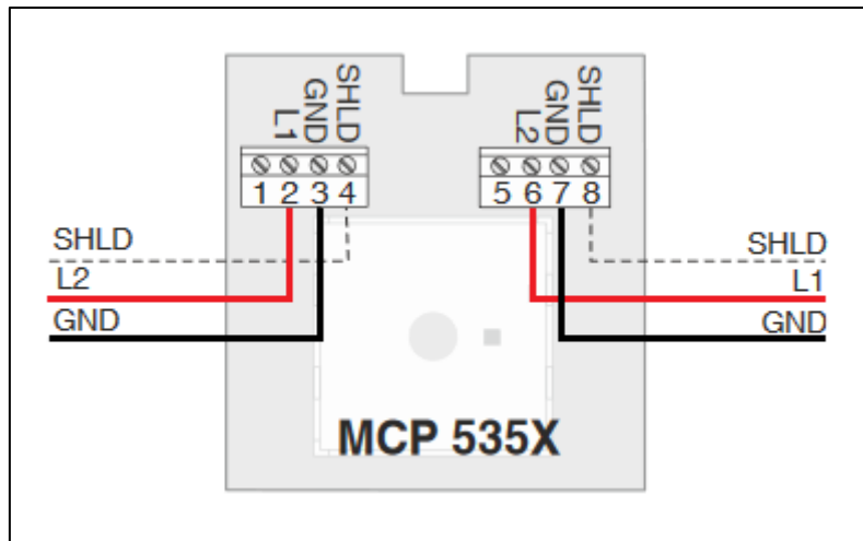
RUČNI JAVLJAČ
